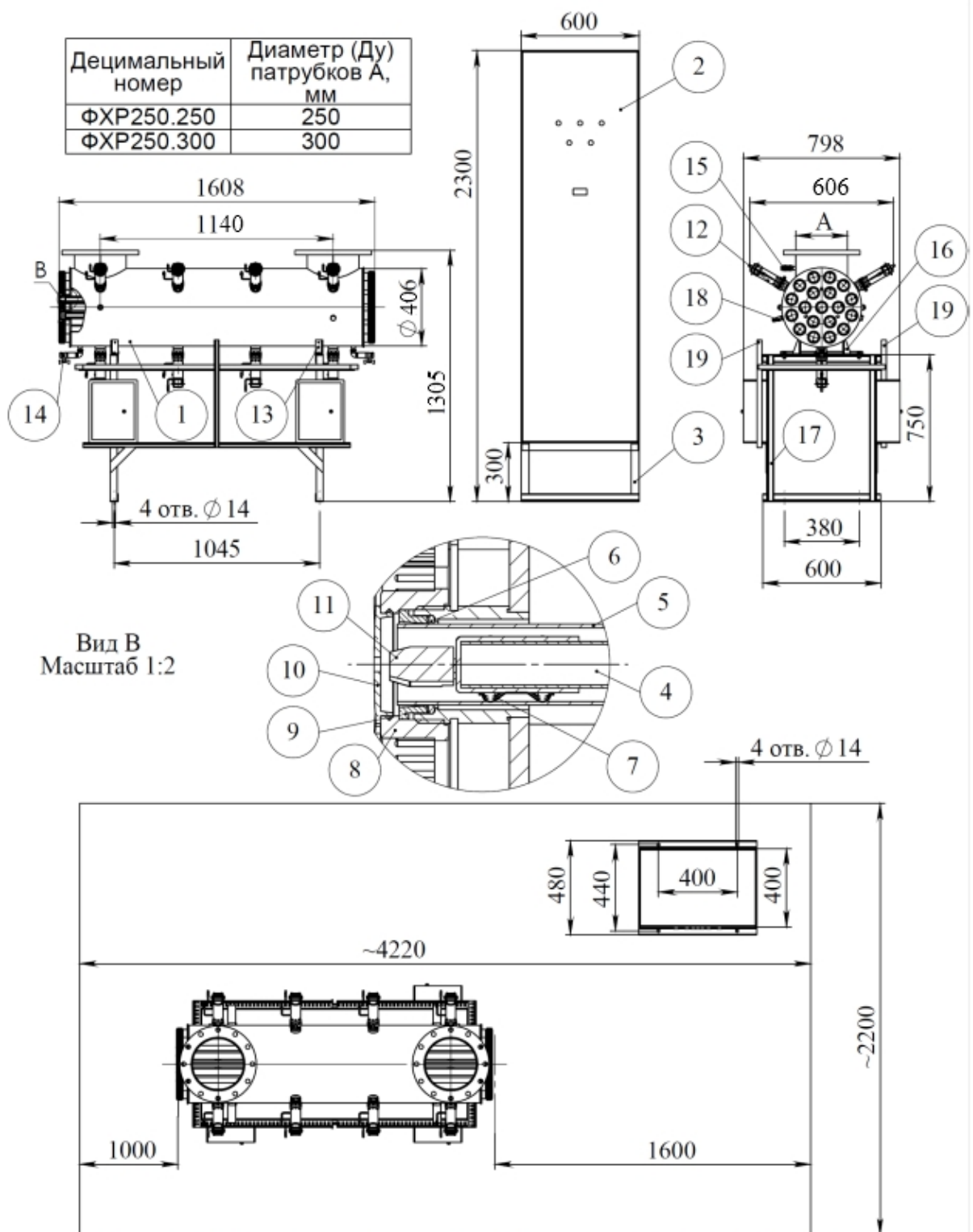
Рис. 1 Общий вид и план размещения установки Лазурь М-250КА
