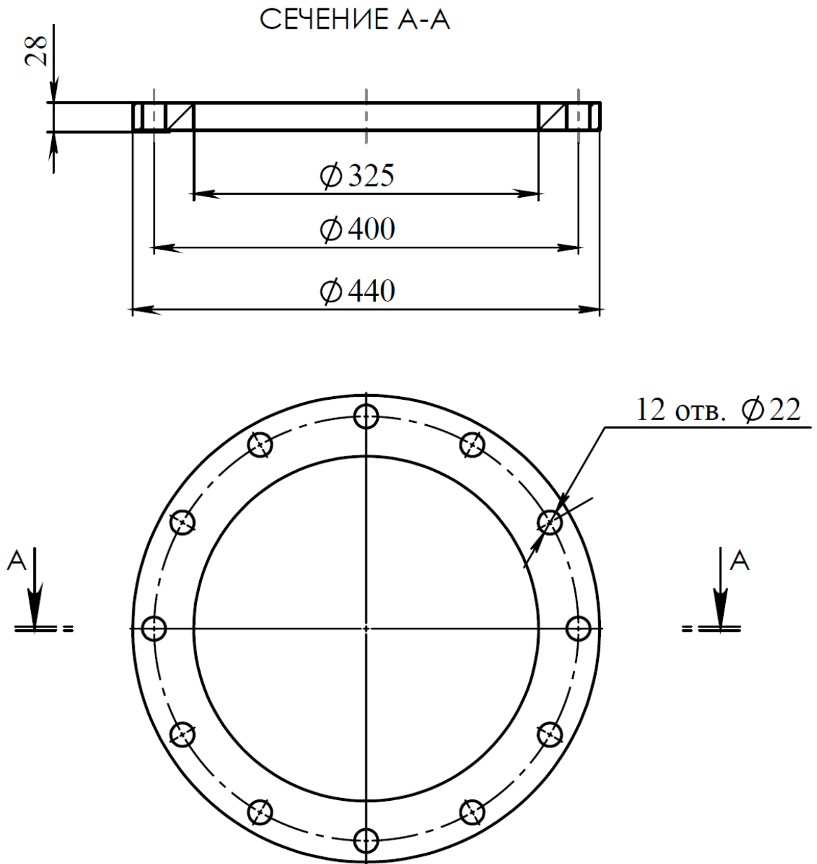
Рис. 3.2 Фланец 1-300-10 ст.12Х18Н10 ГОСТ 12820-80
