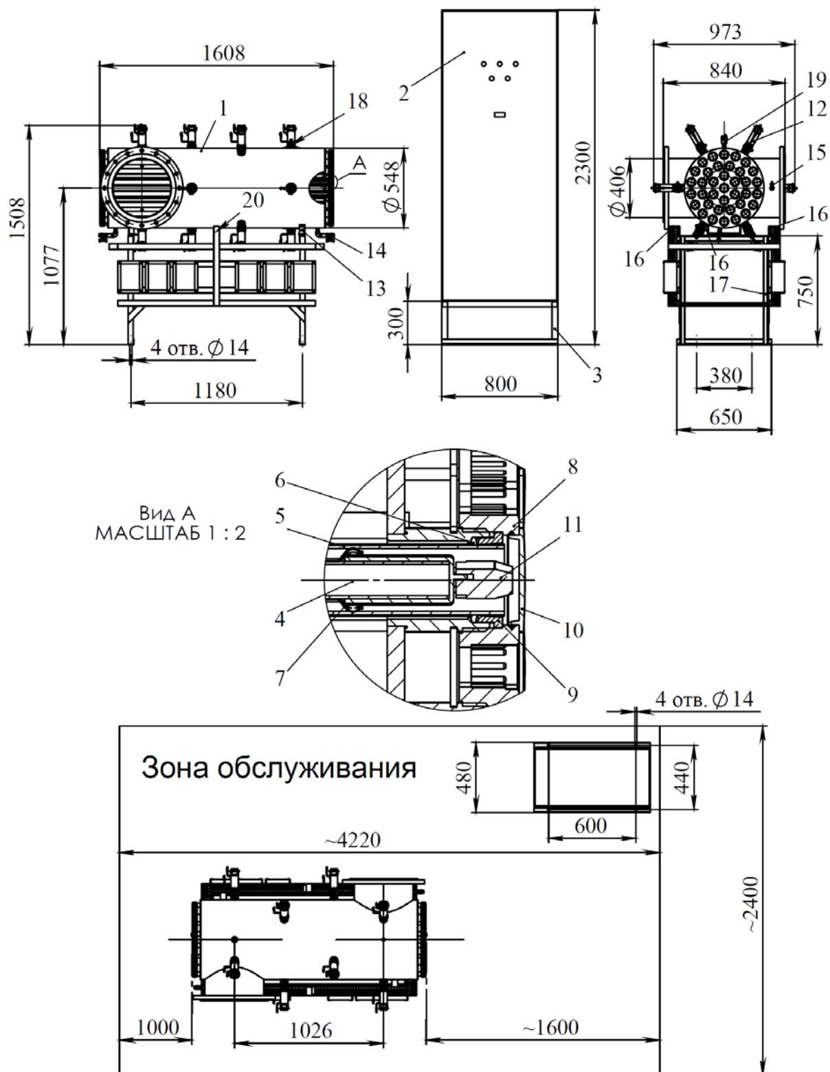
Рис. 1.2 Общий вид и план размещения установки Лазурь М-500.400П 1. Фотохимический реактор 2. Шкаф управления 3. Подставка шкафа управления 4. Ультрафиолетовая лампа 5. Защитная кварцевая трубка 6. Уплотнительное кольцо 7. Распорка пружинная 8. Гайка 9. Нажимное кольцо 10. Заглушка 11. Патрон лампы 12. Ультразвуковой излучатель 13. Клемма заземления 14. Кран для слива воды 15. Кран отбора проб 16. Опора реактора 17. Подставка реактора 18. УФ-датчик 19. Воздухоотводчик 20. Точки ввода электрических кабелей
