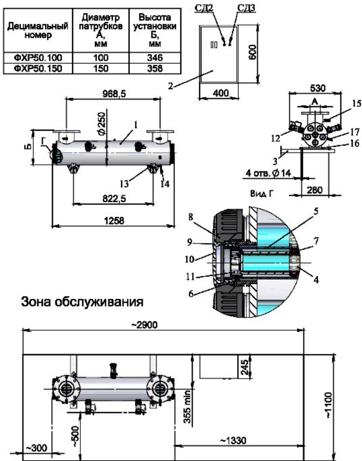
Рис. 1 Общий вид и план размещения установки Лазурь М-50КА
