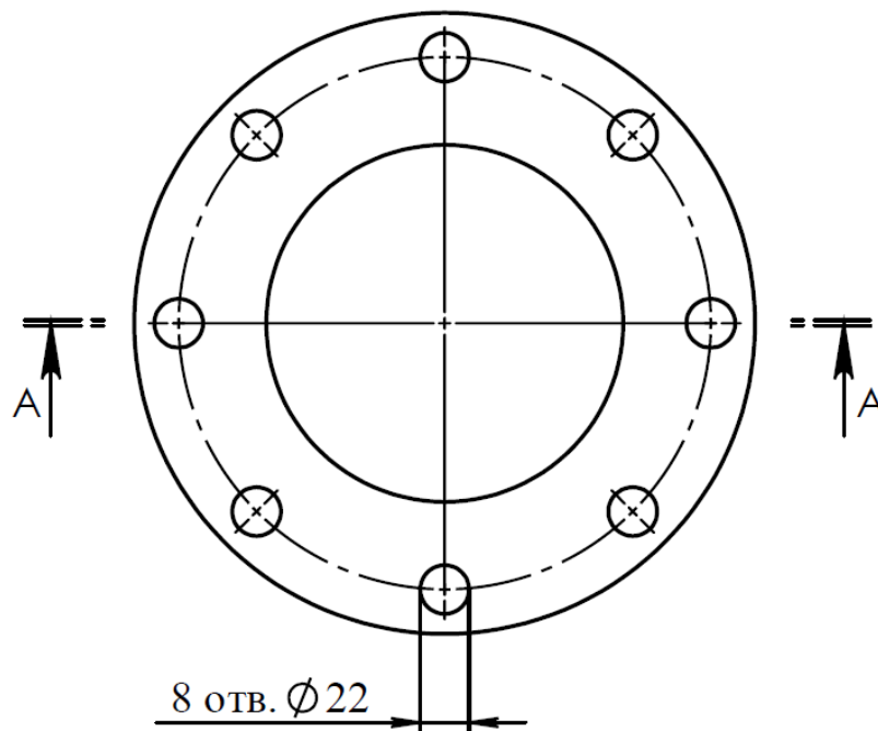
Рис. 3.2 Фланец 1-150-10 ст.12Х18Н10 ГОСТ 12820-80
