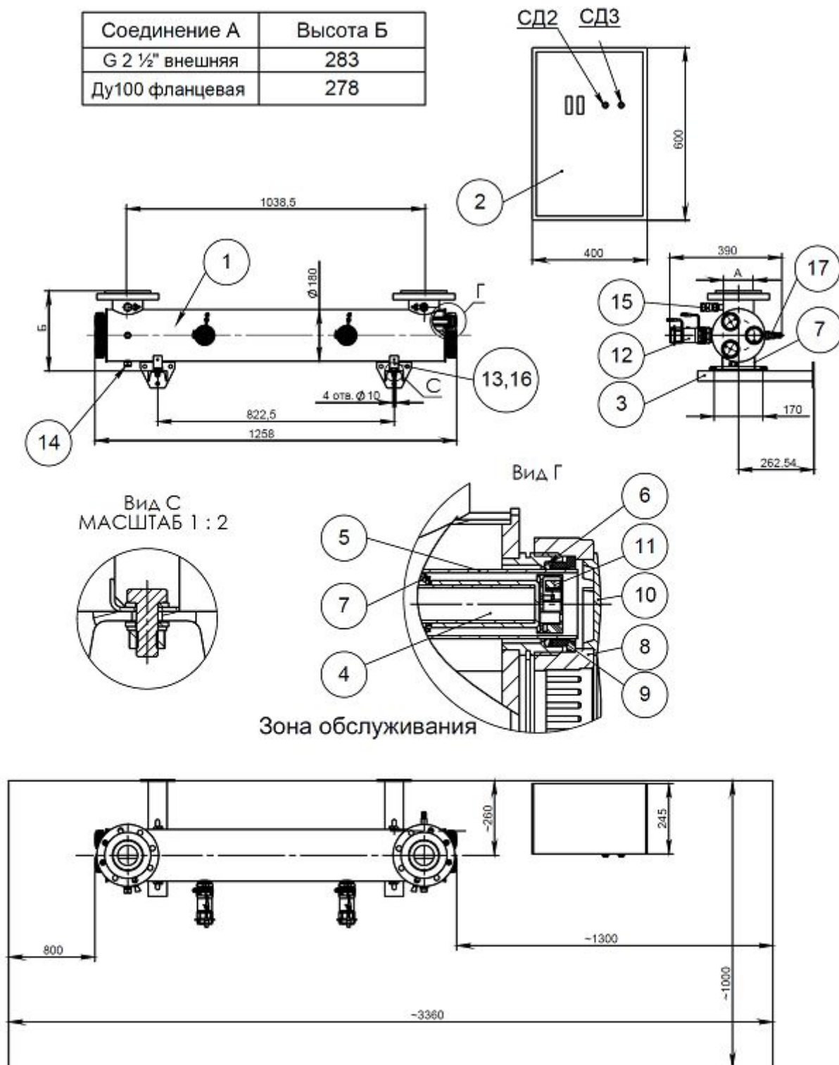
Рис. 1 Общий вид и план размещения установки Лазурь М-30КА
